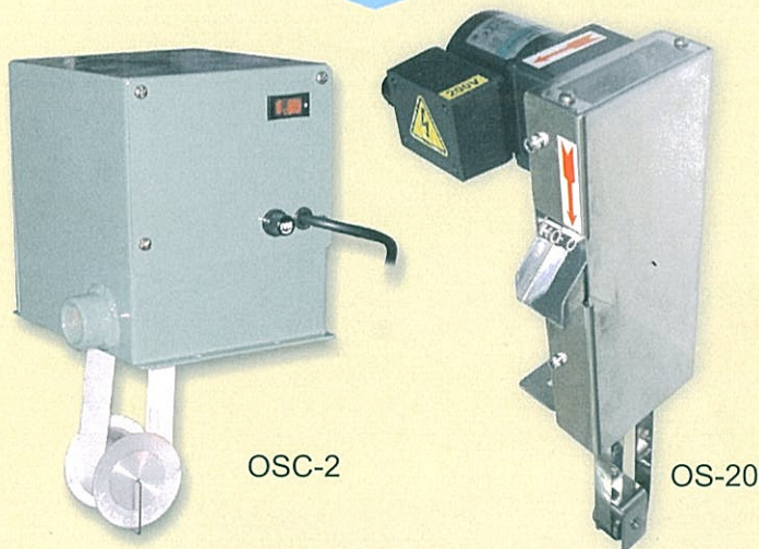
皮帶式油水分離機規格
