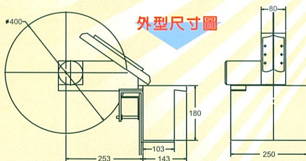
圓板式油水分離機規格
